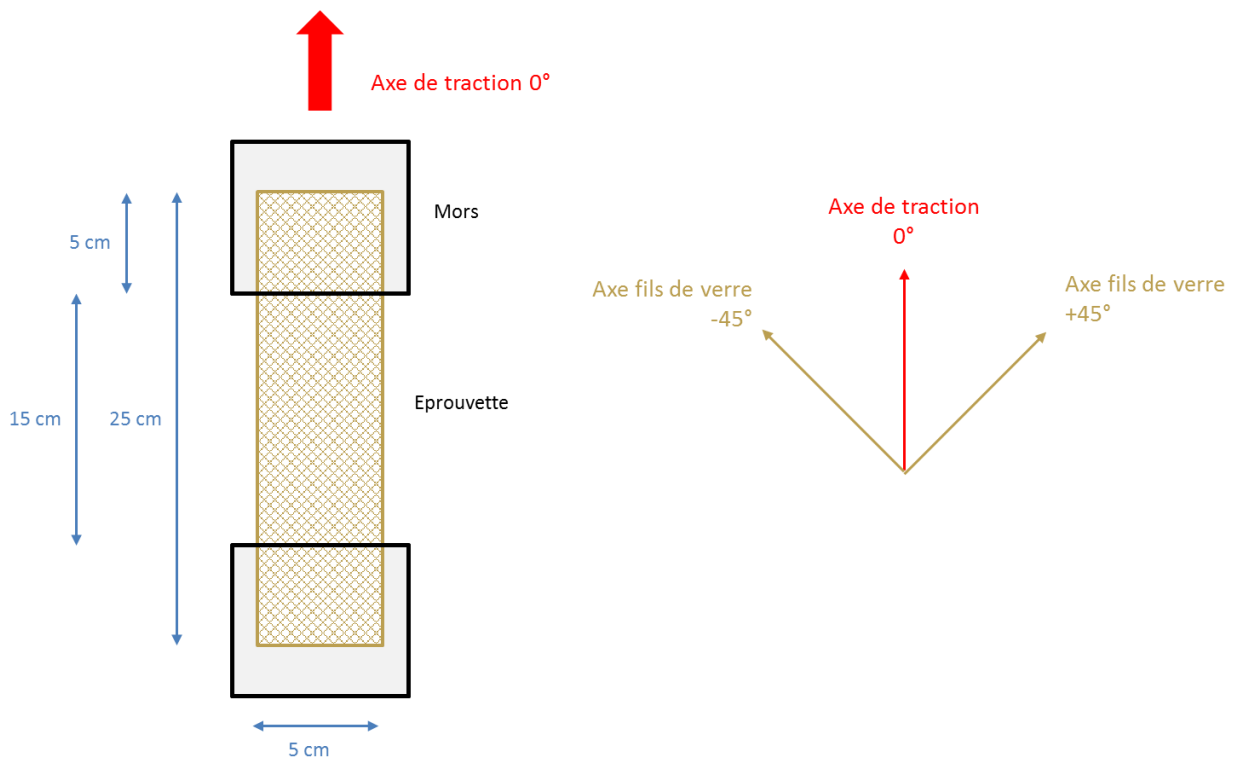
Figure 3 : Exemple de positionnement de l'éprouvette suivant l'axe faible d'un renfort bidiagonal
