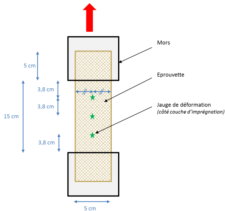
Figure 4 : Exemple de positionnement des jauges de déformation Note : La tolérance de positionnement est de + ou – 5 mm.
